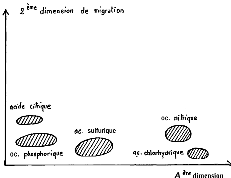
Flg. 13- Analyse qualitative des acides organiques par chromatographie
